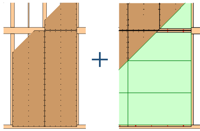
構造用合板
