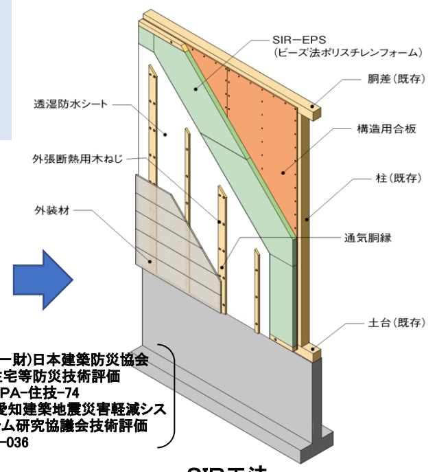
SIR工法
