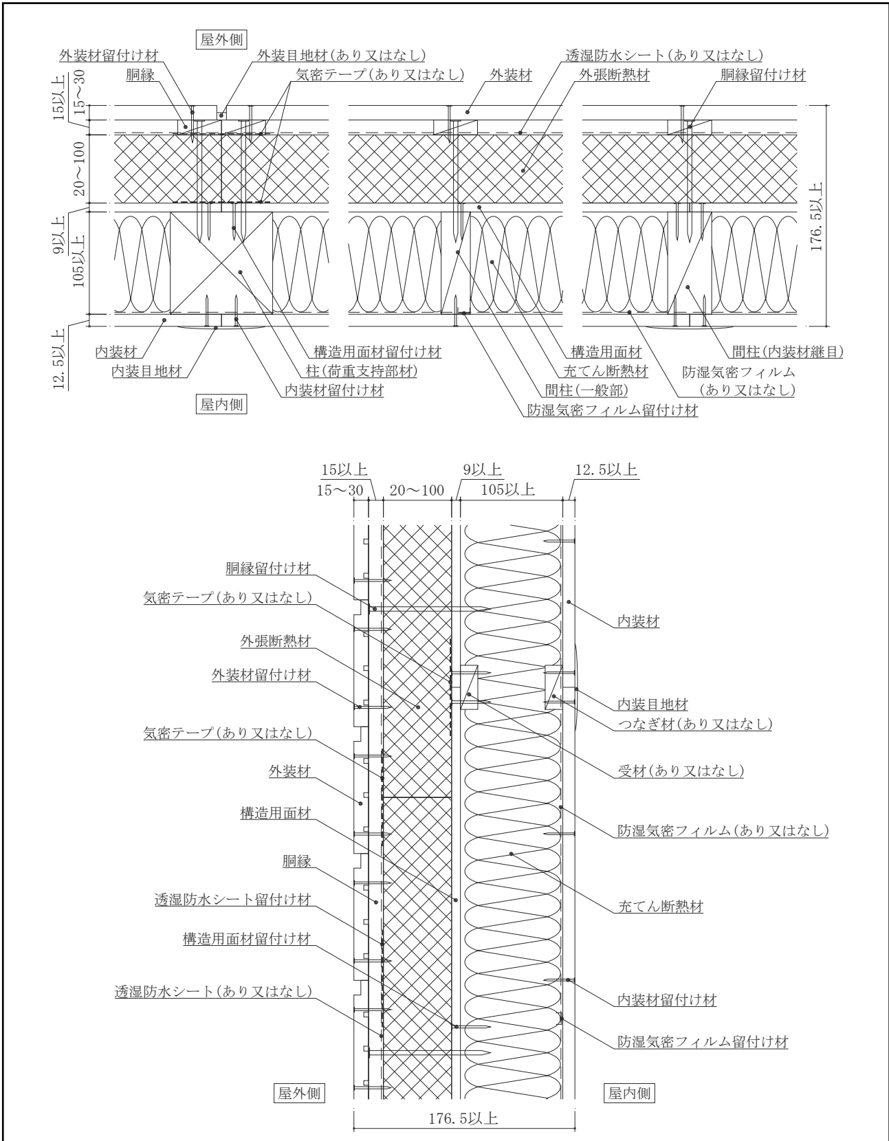
図2 構造説明図
