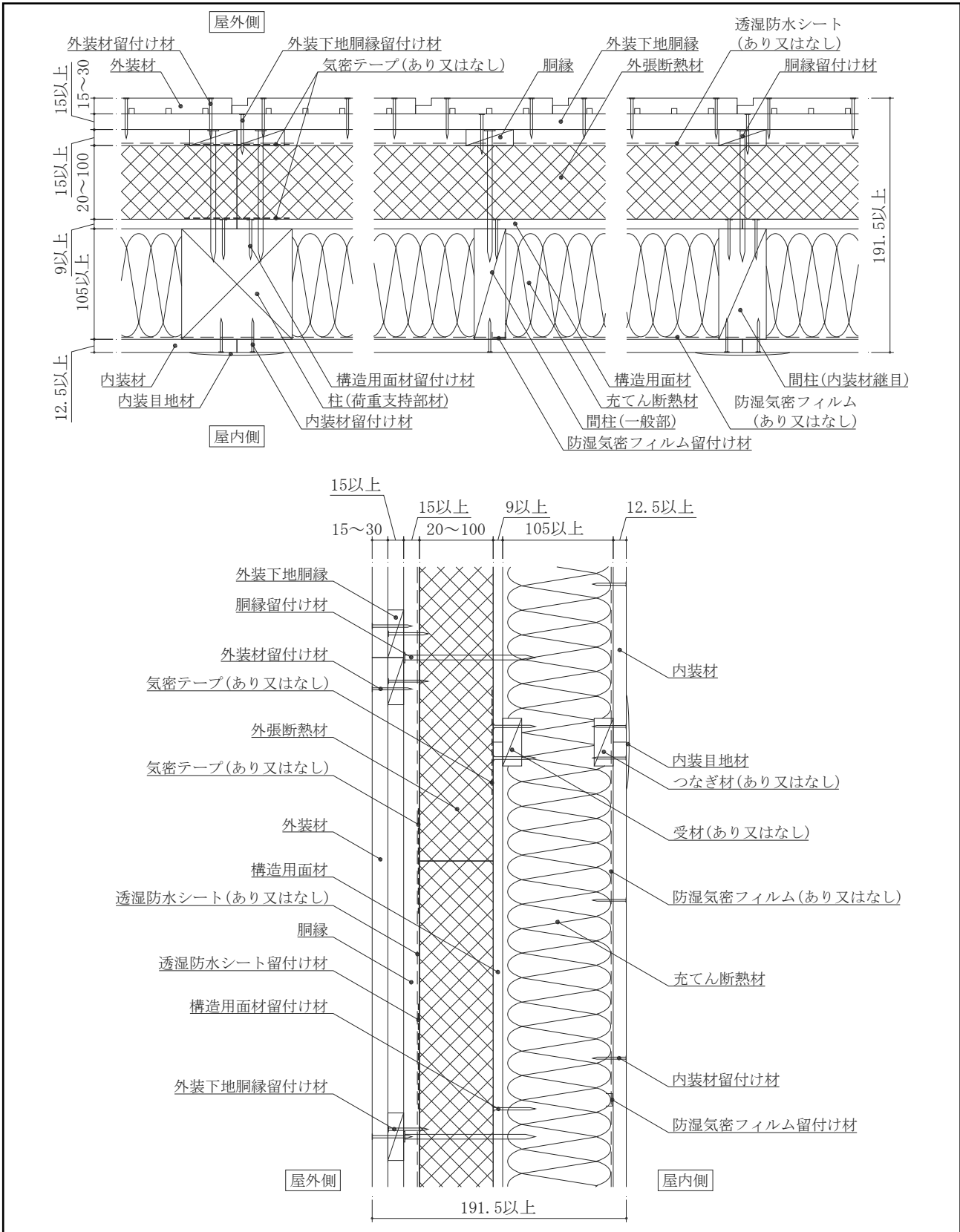
図6 構造説明図
