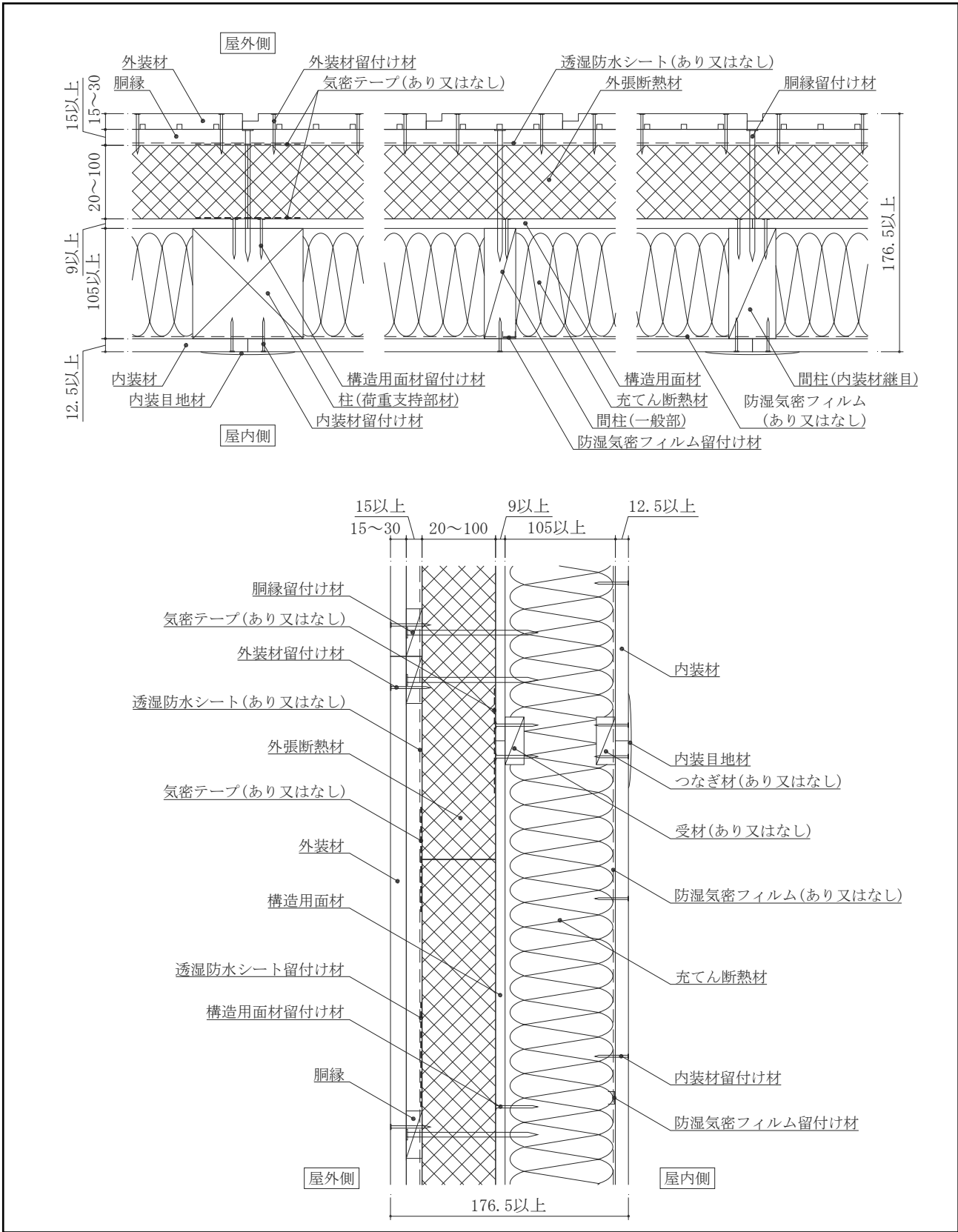
図4 構造説明図
